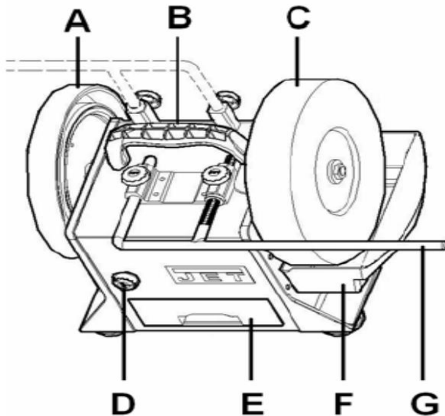
А. Съёмный кожаный шлифовальный круг; В. Ручка; С. Шлифовальный круг; D. Регулятор частоты вращения полировального круга; Е. Ящик для инструментов; F. Ёмкость для воды; G. Стандартная направляющая
